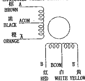
【电机接线图 WIRING DIAGRAM】
