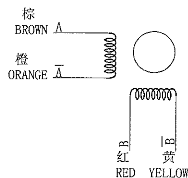
【电机接线图 WIRING DIAGRAM】
